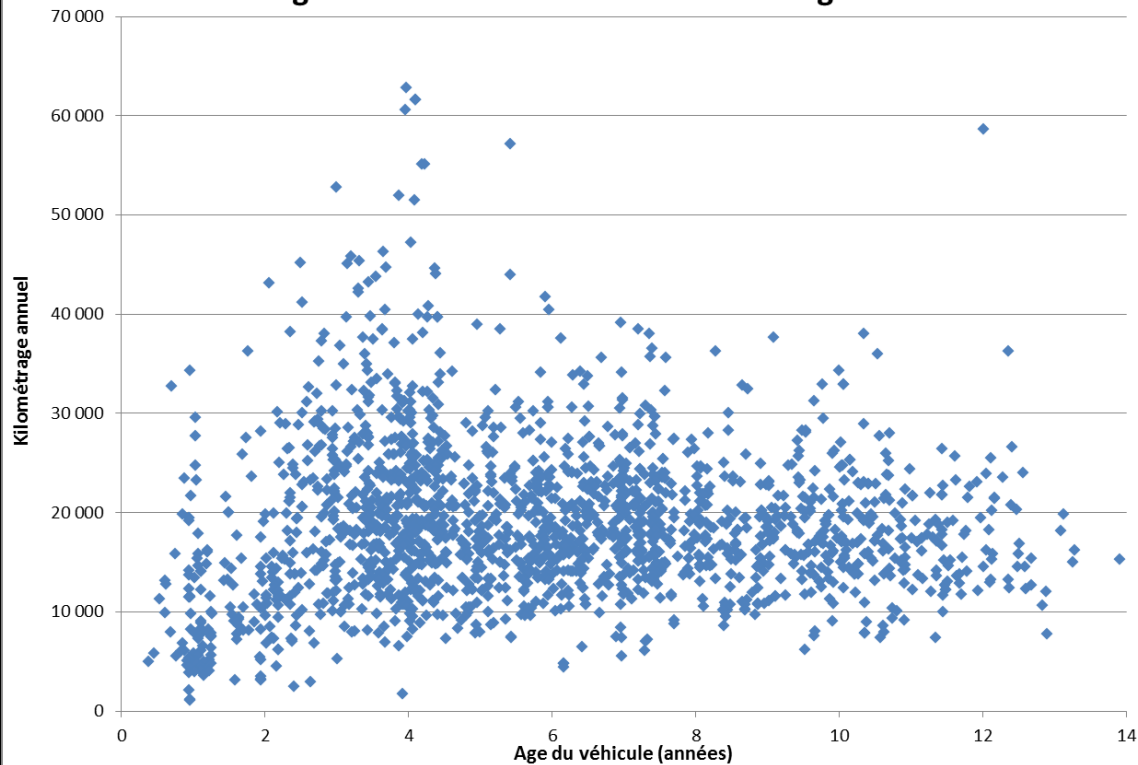
Kilométrage annuel constaté en fonction de l'âge du véhicule
